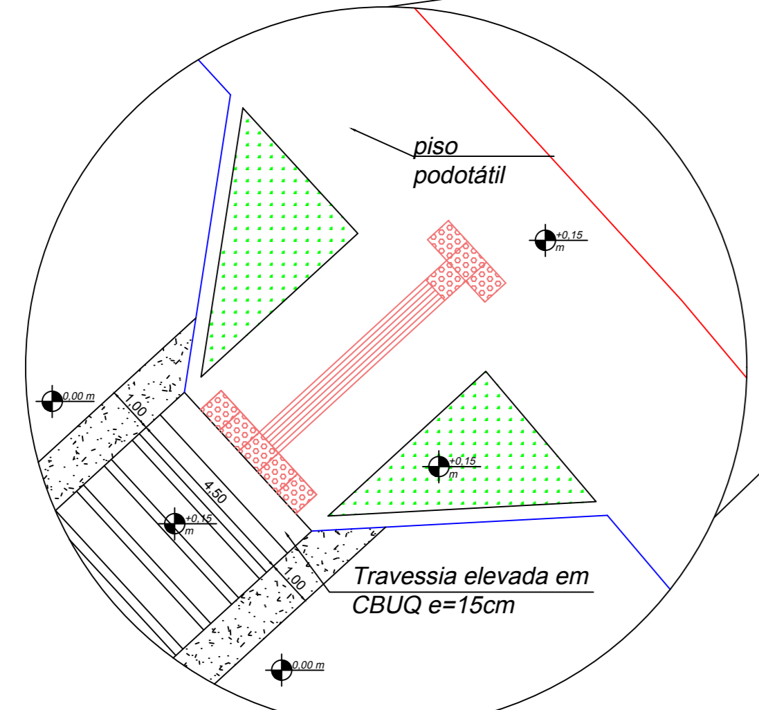
Detalhe 2 - CT - Canteiro de Travessia
