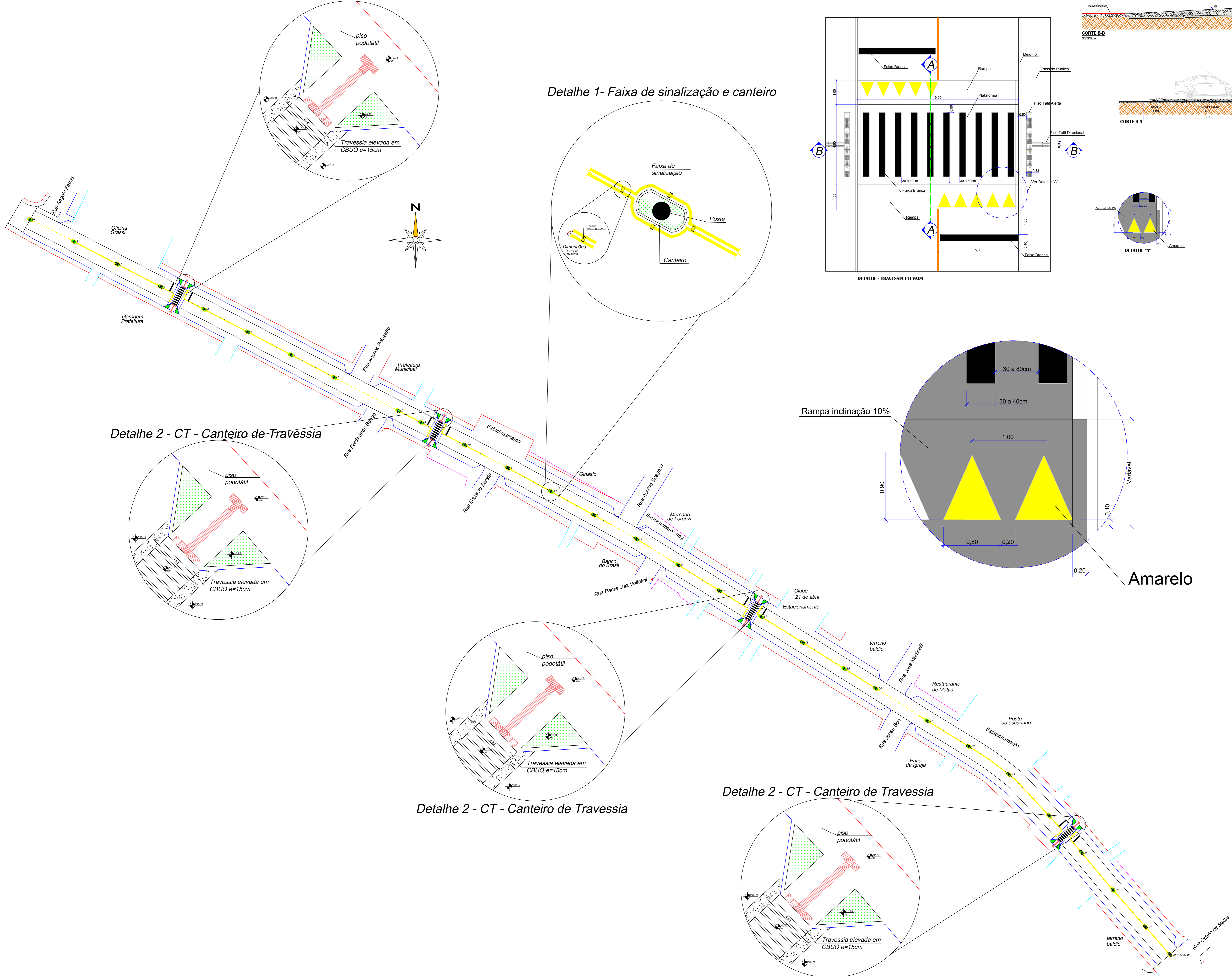
Detalhe 2 - CT - Canteiro de Travessia
