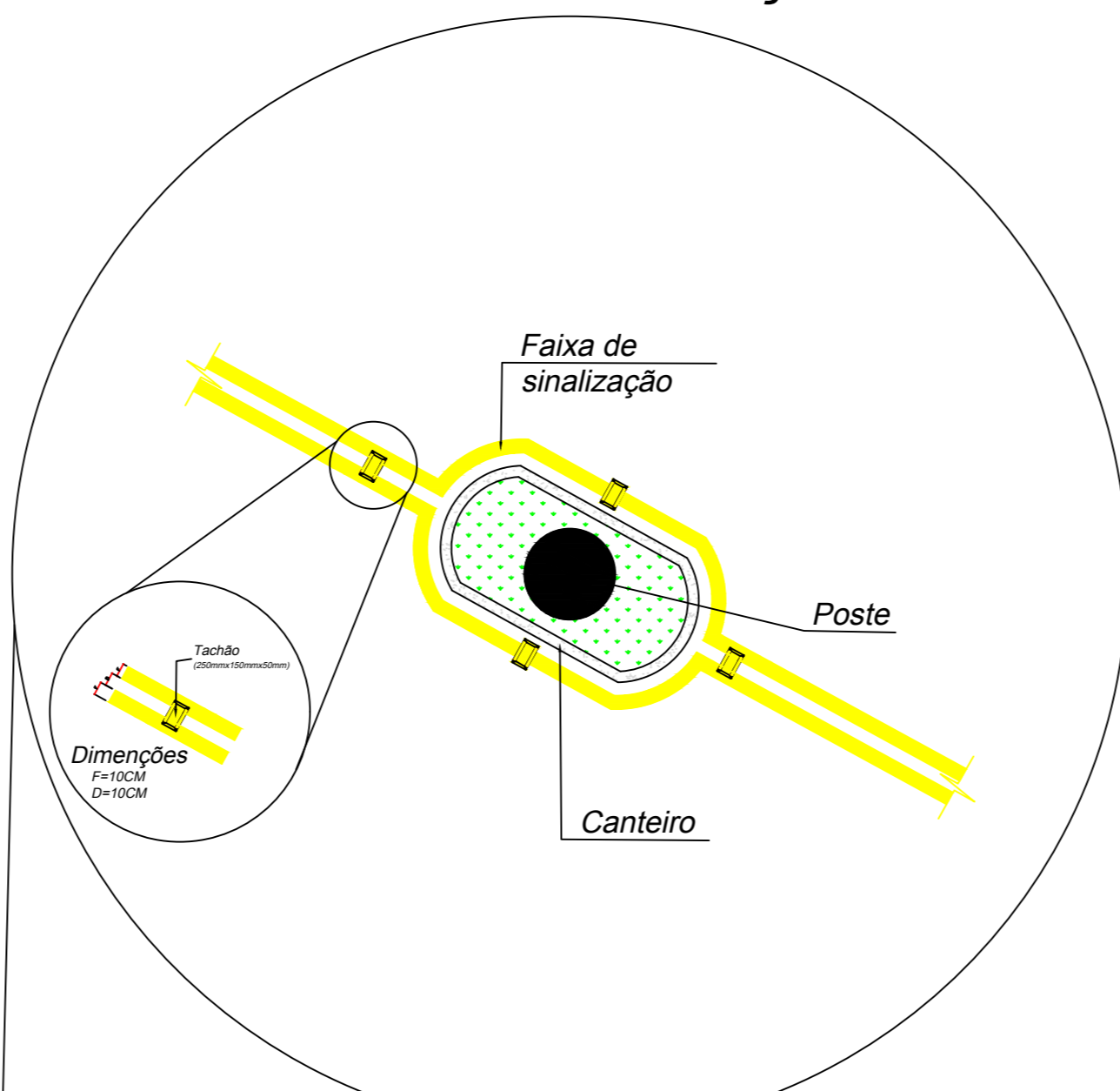
Detalhe 1- Faixa de sinalização e canteiro
