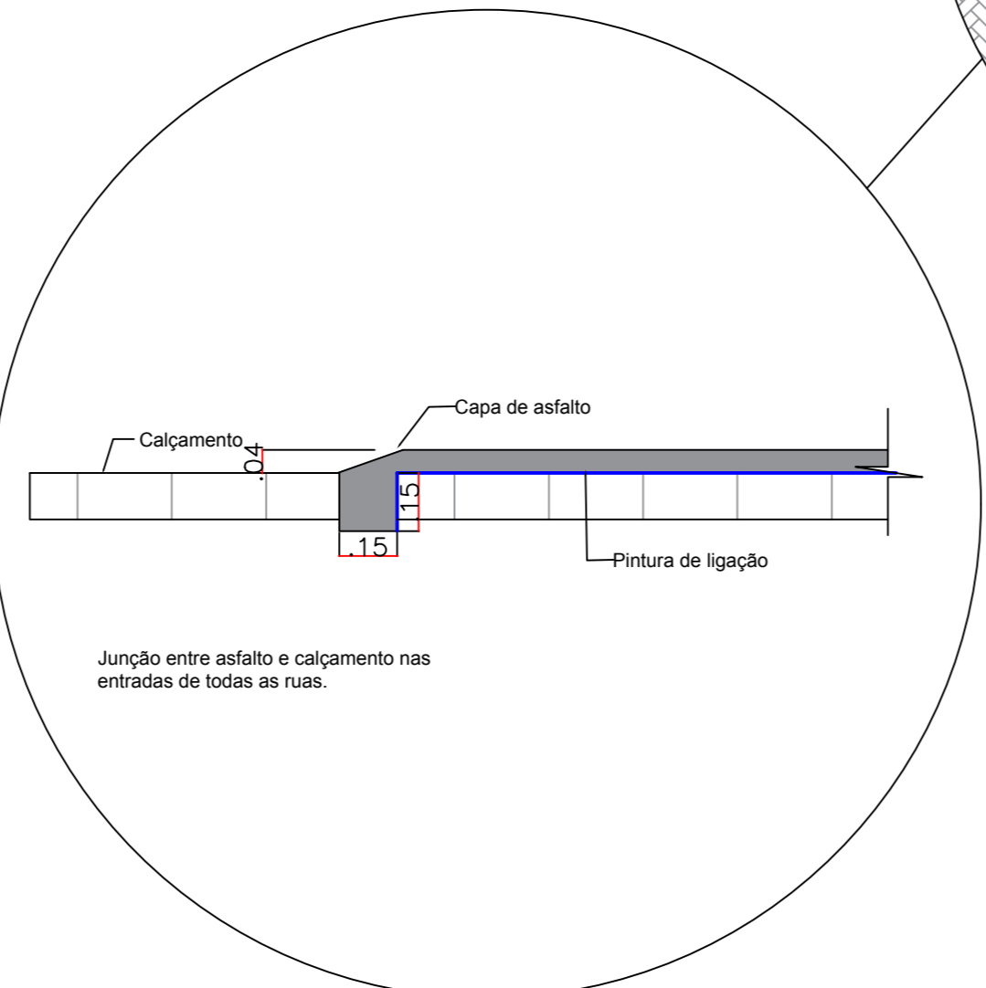
Detalhe 4 - Extensão da capa de asfalto
