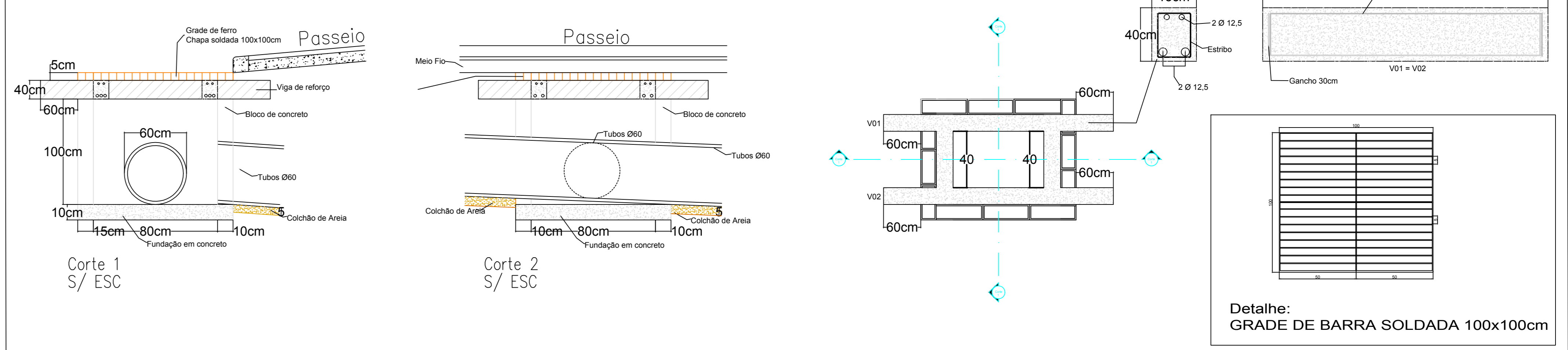
Detalhe 5: Caixas Coletoras
