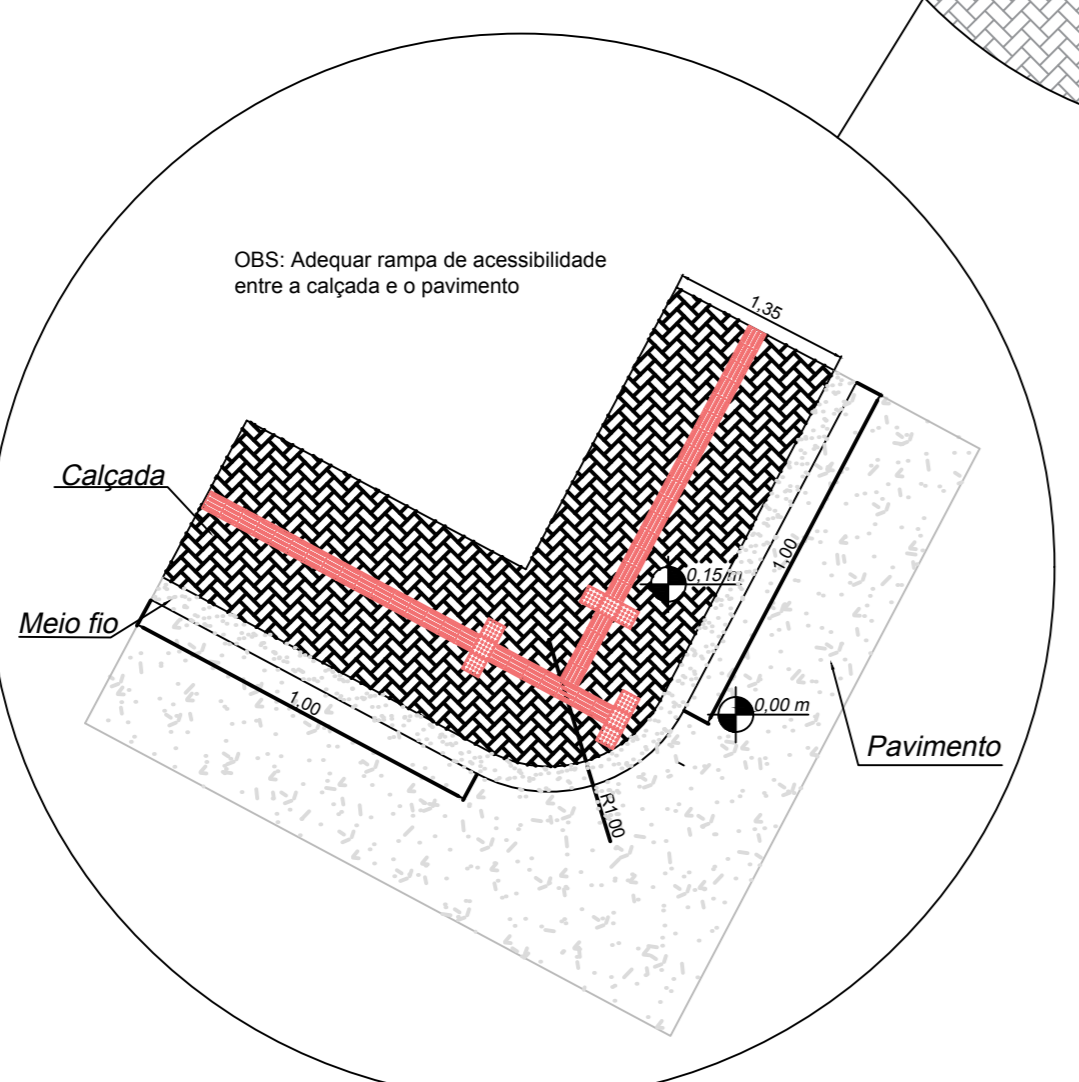
Detalhe 6 - Calçadas das Esquinas (modelo a ser adequado)
