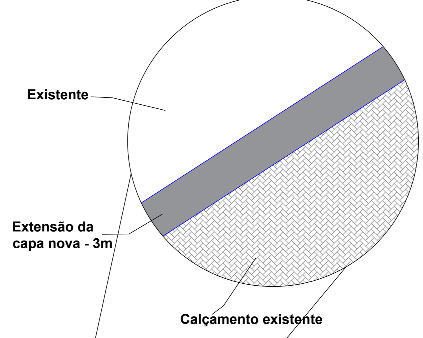
Detalhe 3- Extensão da capa de asfalto
