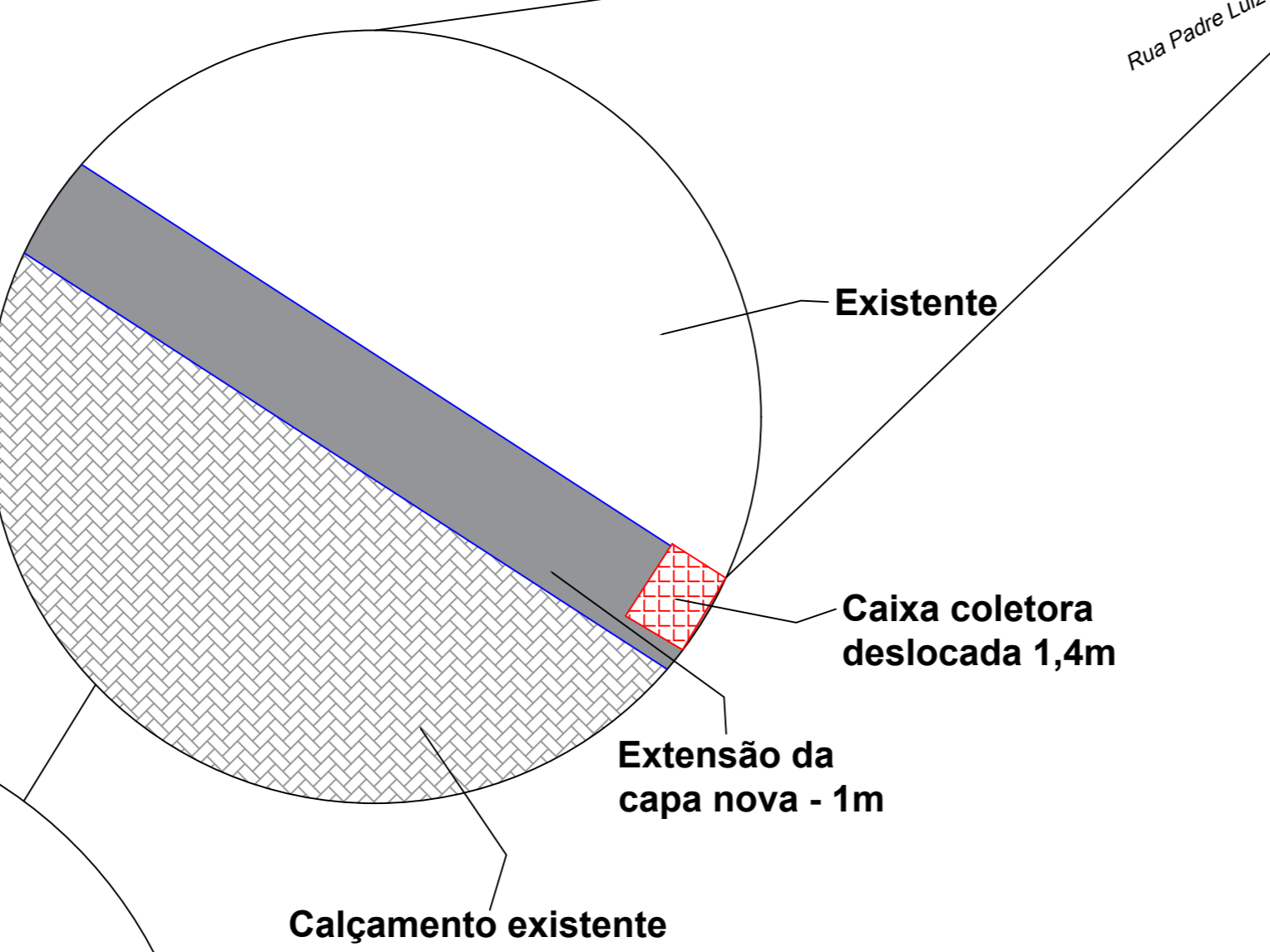
Detalhe 3- Extensão da capa de asfalto
