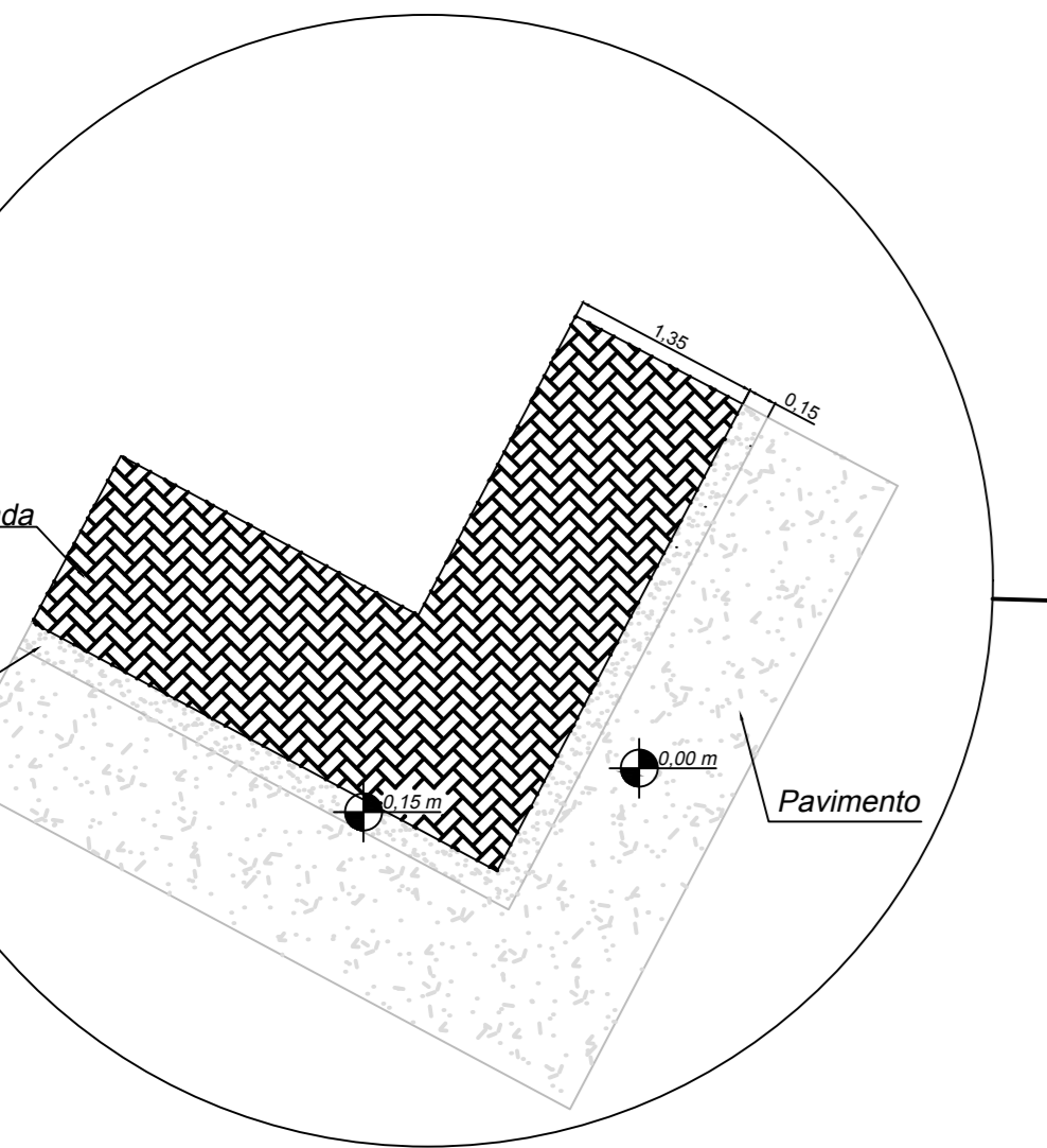
Detalhe 6 - Calçadas das Esquinas (Existente)
