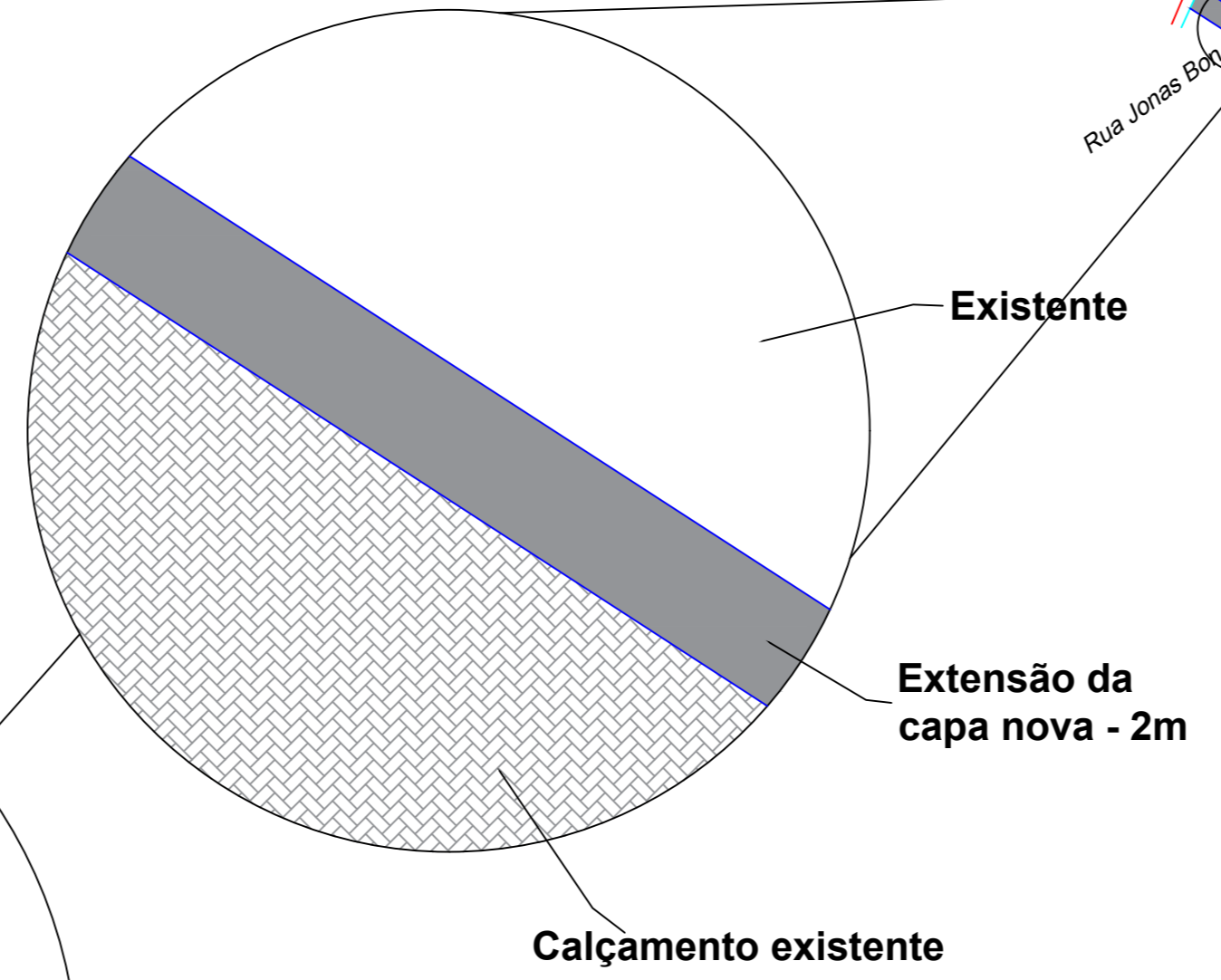
Detalhe 3- Extensão da capa de asfalto
