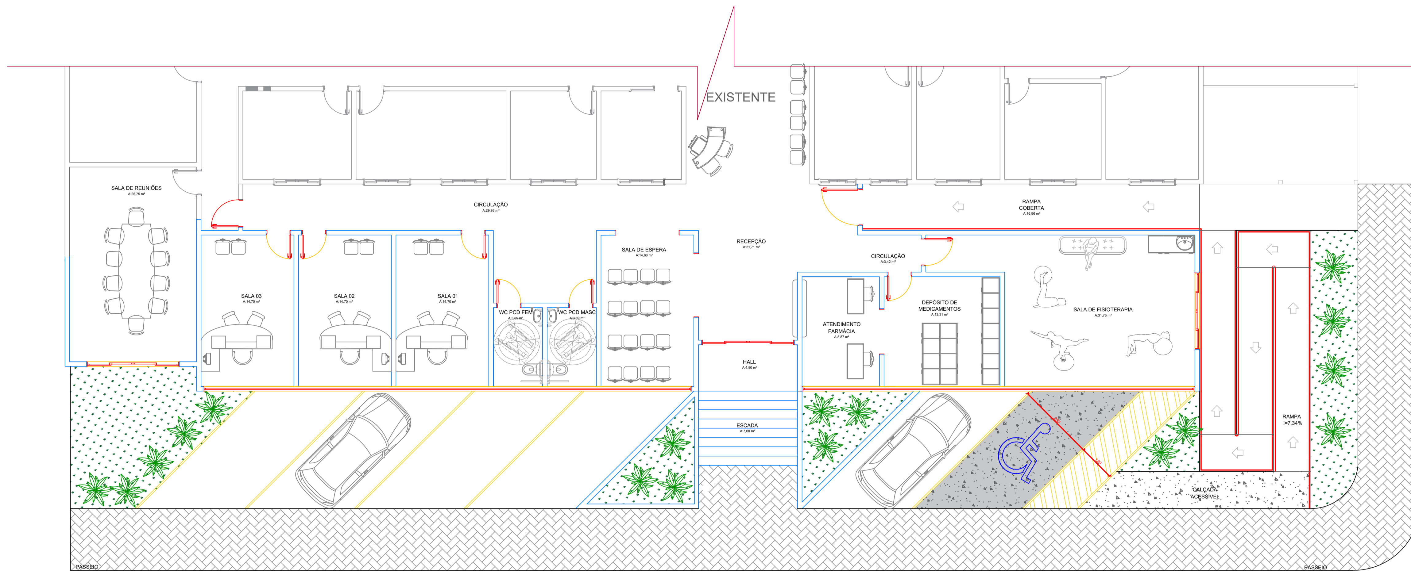
PLANTA BAIXA DE LAYOUT ESC.: 1:75
