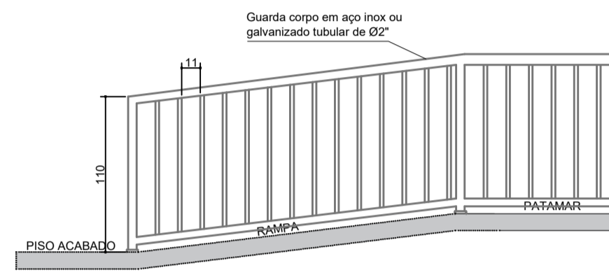
DETALHE - GUARDA CORPO RAMPA S/ESC
