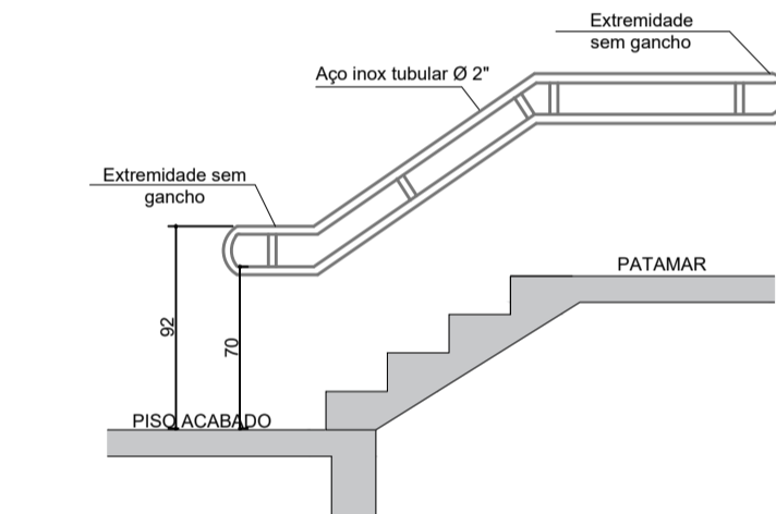
DETALHE - CORRIMÃO ESCADA S/ESC
