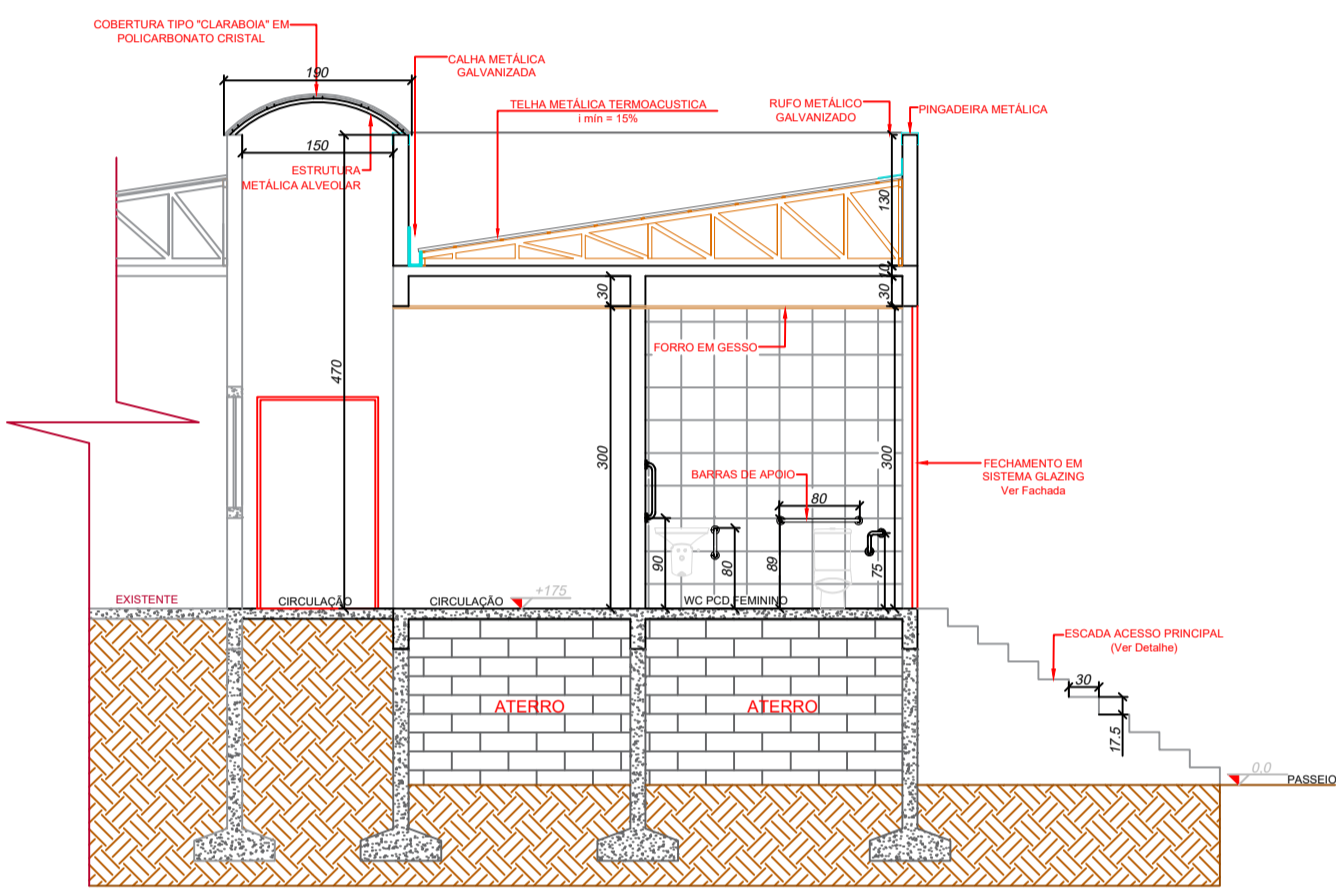
CORTE BB ESC.: 1/75
