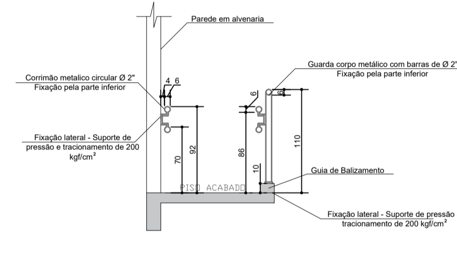
DETALHE - CORTE ESQUEMÁTICO GUARDA CORPO E CORRIMÃO S/ESC
