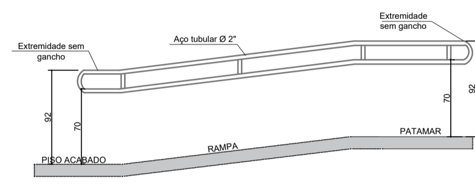
DETALHE - CORRIMÃO RAMPA S/ESC
